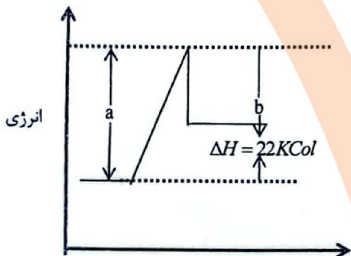
پیشرفت واکنش
